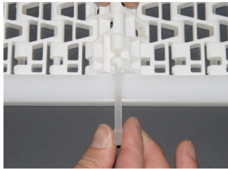
Inserte la varilla
