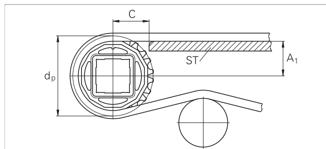
Piñón de una pieza (sólido)
